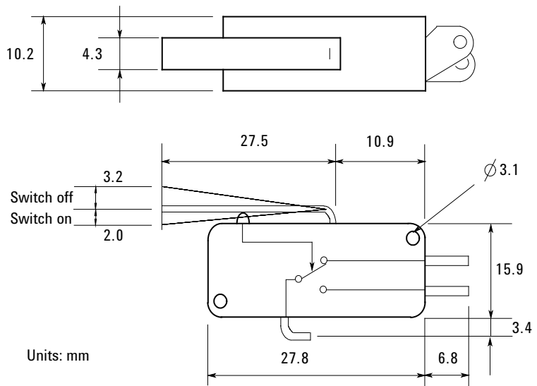
Figure 3-14 インターロック・スイッチの寸法 (Agilent 部品番号 3101-3241)
