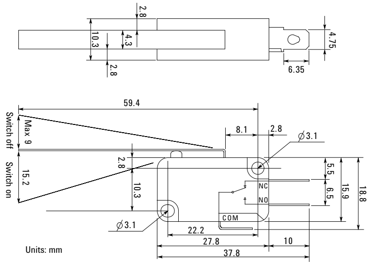
Figure 3-13 インターロック・スイッチの寸法 (Agilent 部品番号 3101-0302)
