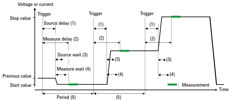
Figure 6-1 ソース出力と測定タイミング、掃引出力例
