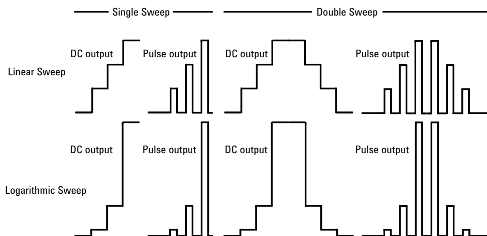
Figure 6-3 様々な掃引出力
